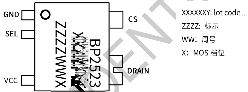
图 2 管脚封装图
